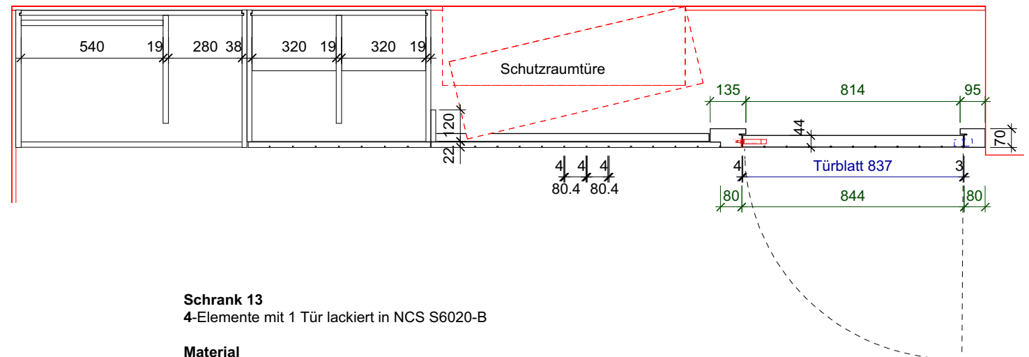
B-B
